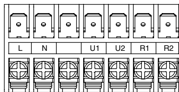
Панель роз'ємів 7-полюсних
