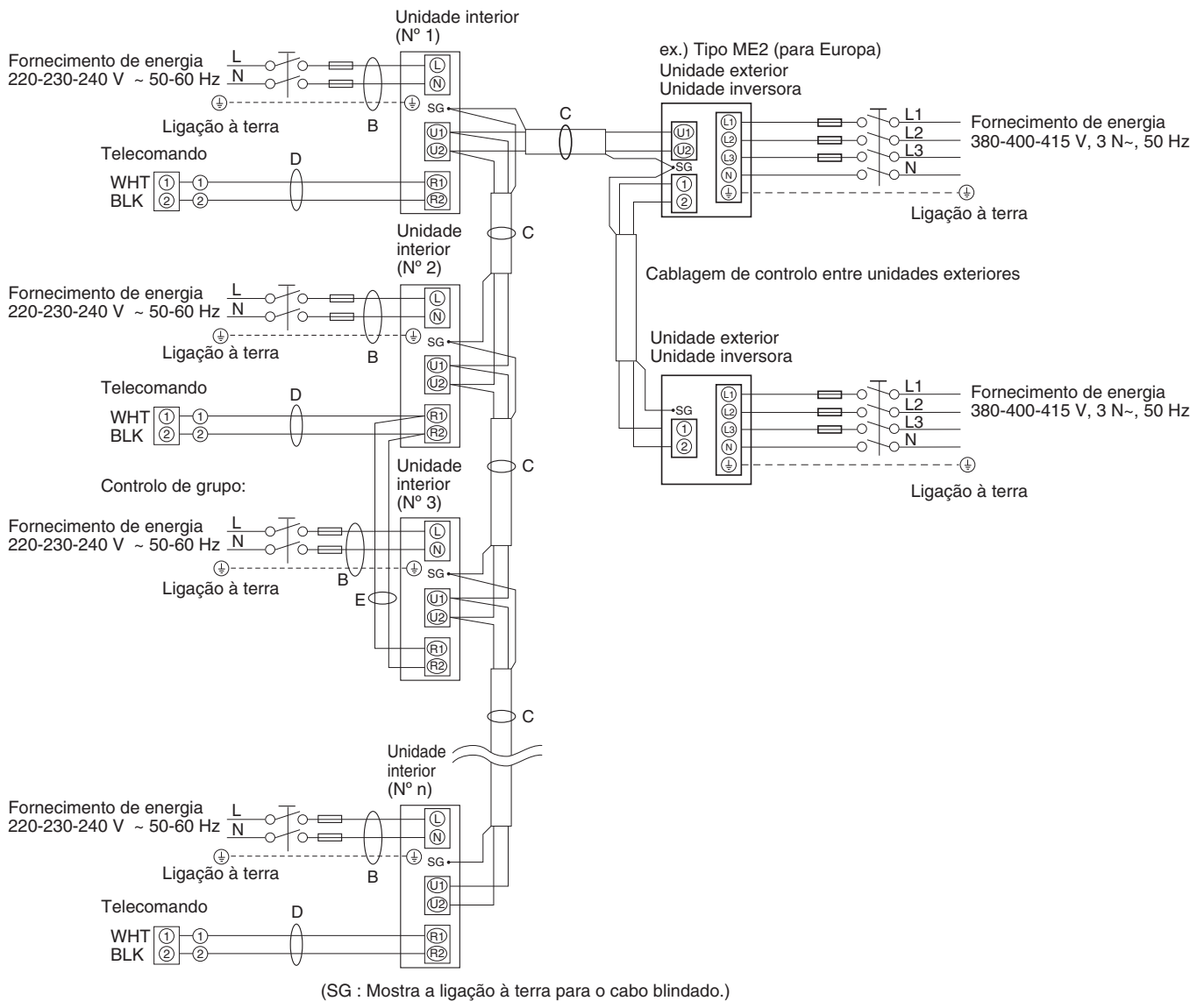
Quadro de terminais 7P
