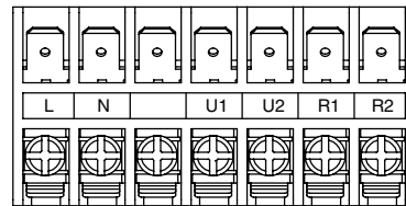
Alimentation Câblage de commande inter-unités Câblage de télécommande
