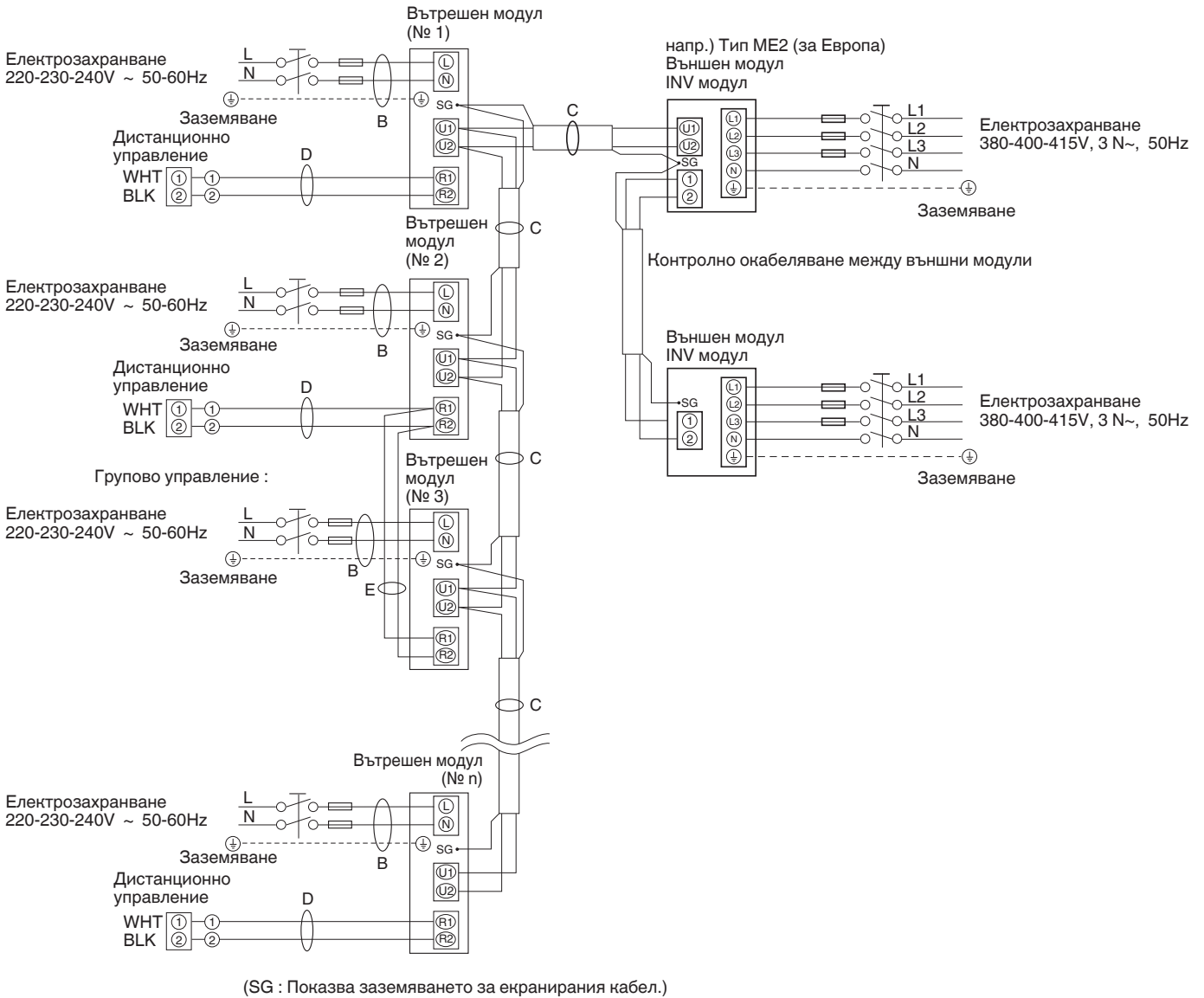
Клемно табло 7P
